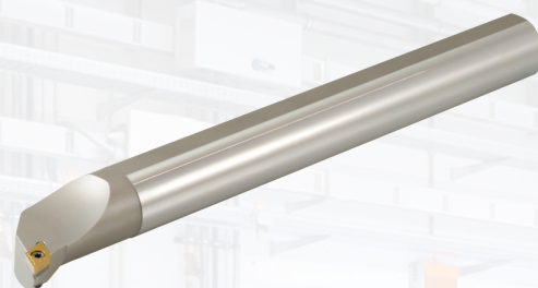
Indvendige borestænger til DC.. 0702.. platter
